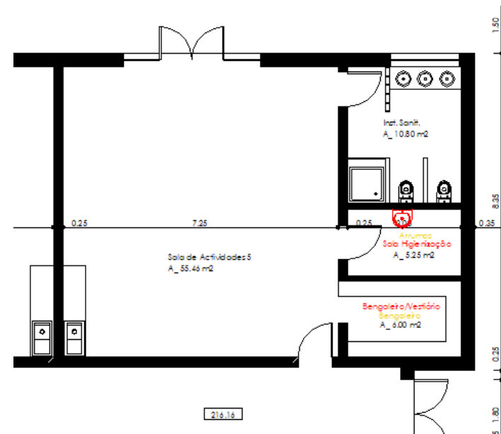
Fig. 12 – Alterações a realizar na sala de actividades 5.
