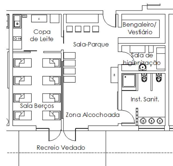
Fig. 13 – Divisão da Sala de Actividades 6.
