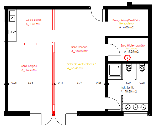
Fig. 14 – Alterações da Sala de Actividades 6.
